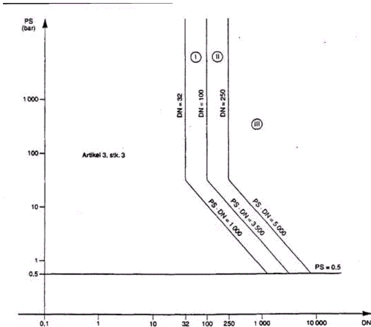
Diagram 7 - Rørsystemer omhandlet i artikel 3, stk 1.3, litra a), andet led. Gælder for rørsystemer indeholdende damptryk over 0,5 bar og ikke farlig (Gr.2) fluida.
